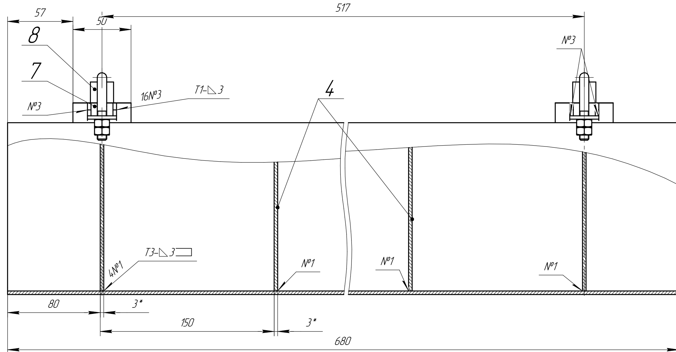
Дет. поз. 2 (1:1)
