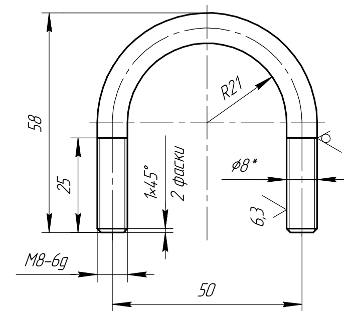
Дет. поз. 6 (1:1)
