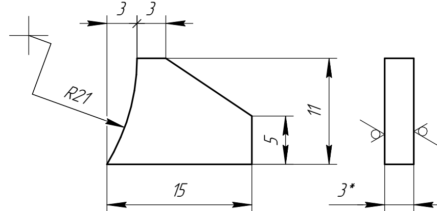
Дет. поз. 5 (2,5:1)
