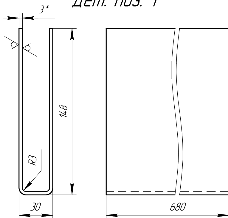
Дет. поз. 1
