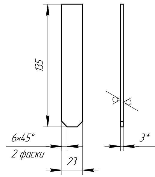
Дет. поз. 4 (1:2,5)
