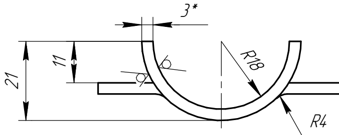
Дет. поз. 2 (1:1)
