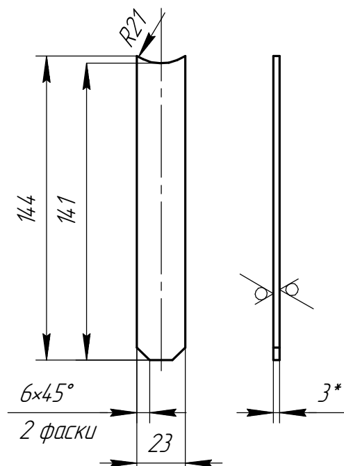
Дет. поз. 3 (1:2,5)
